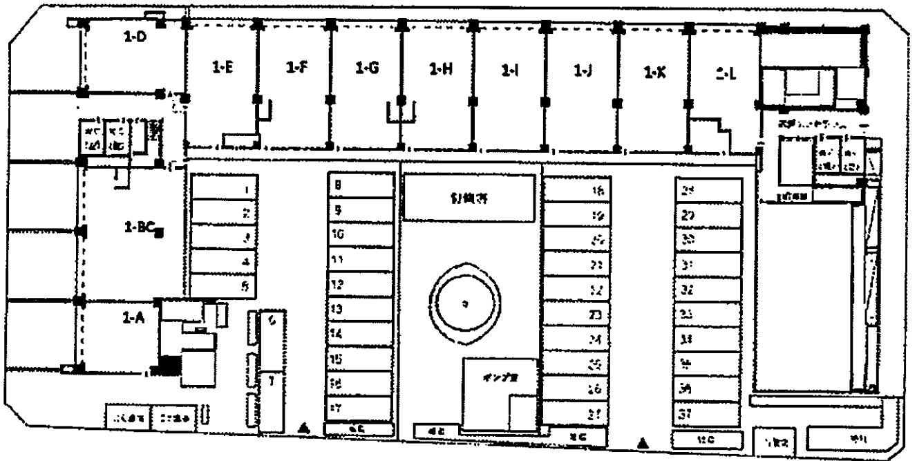
根岸駅前ビル配器図・1F平面図
